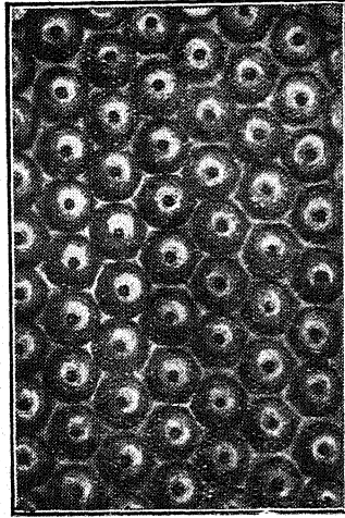
चित्र १६६—घरेलू मक्खी की असंख्य आंखें, अणुवीक्षण द्वारा देखी गयीं।
